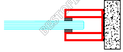
DUVAR BAŞLANGICI
